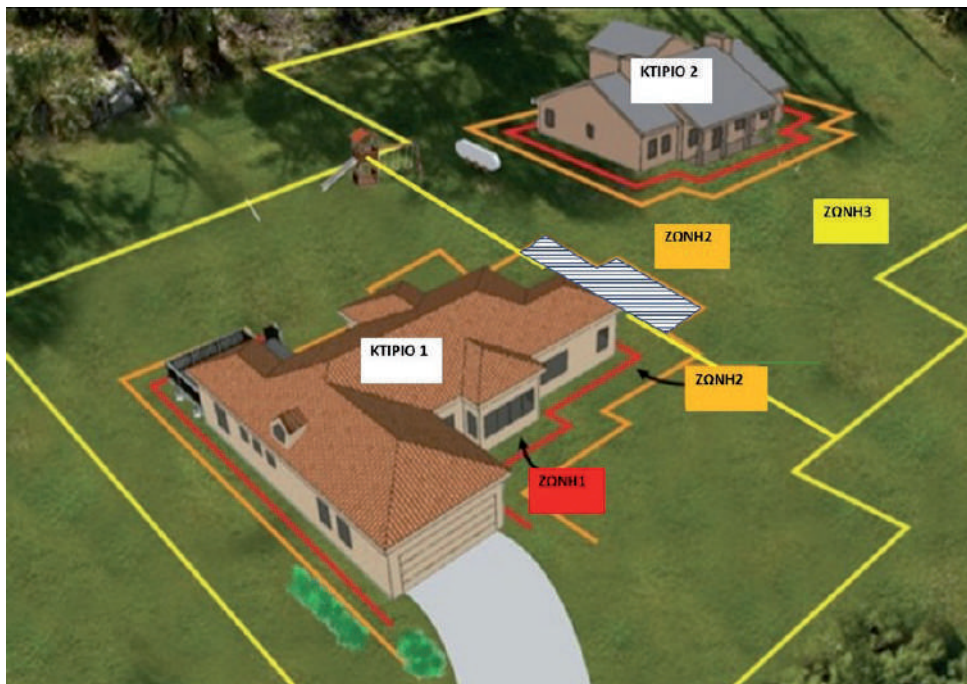
β. Το ακίνητο με το κτίριο 1 δεν έχει επαρκές πλάτος για πλήρη ανάπτυξη της ζώνης 2 στα ανατολικά του και τμήμα αυτής (με διαγράμμιση) εμπίπτει εντός της όμορης ιδιοκτησίας, η οποία στη θέση αυτή βάσει των διαμορφώσεων των ζωνών προστασίας, θα μπορούσε να εφαρμόζει τις προϋποθέσεις της ζώνης 3. Η δημιουργία στη θέση αυτή μίας ζώνης 3, αυξάνει τον κίνδυνο μετάδοσης της πυρκαγιάς στο ακίνητο με το κτίριο 1. Ως εκ τούτου, το ακίνητο 2 οφείλει στο τμήμα της επικάλυψης, να διαβαθμίσει τη φύτευσή του με τέτοιο τρόπο ώστε να ανταποκρίνεται στις απαιτήσεις της ζώνης 2.
